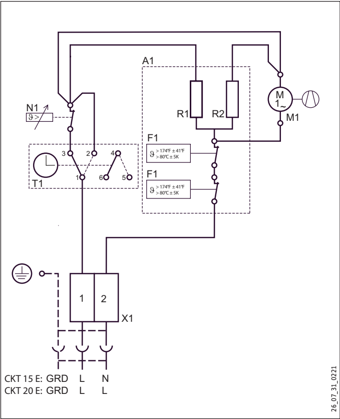
14.3 Plano eléctrico CKT 15 E / CKT 20 E
