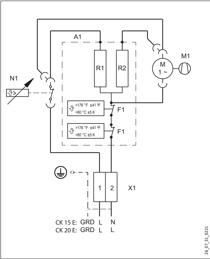
14.2 Plano eléctrico CK 15 E / CK 20 E
